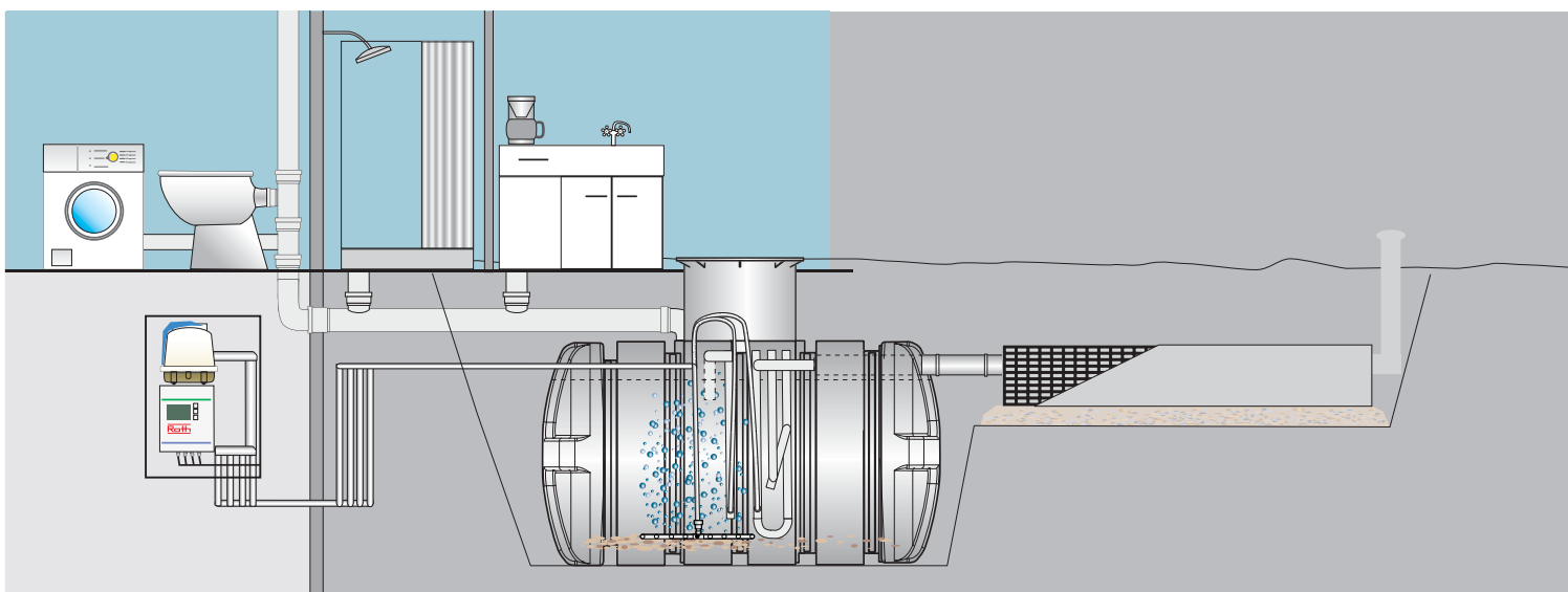
Využití dešťové vody
